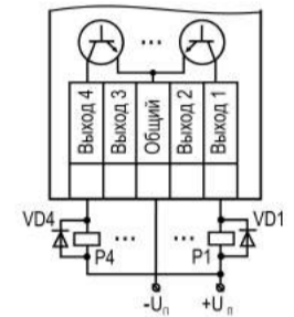
Рисунок 10 – Схемы подключения нагрузок к ВЭ
