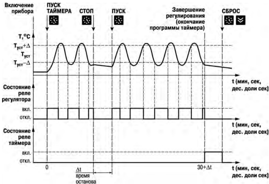
Рисунок 4.1 – График регулирования температуры по программе таймера
