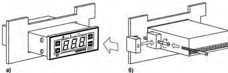
Рисунок 6.1 – Монтаж прибора
