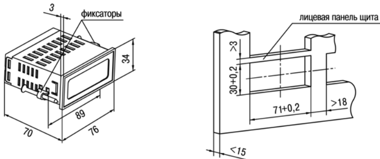
Рисунок А.1 – Габаритные и установочные размеры TPM501
