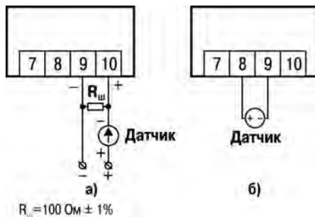
Рисунок 6.4 – Схема подключения датчиков с выходным сигналом тока (а) и напряжения (б)
