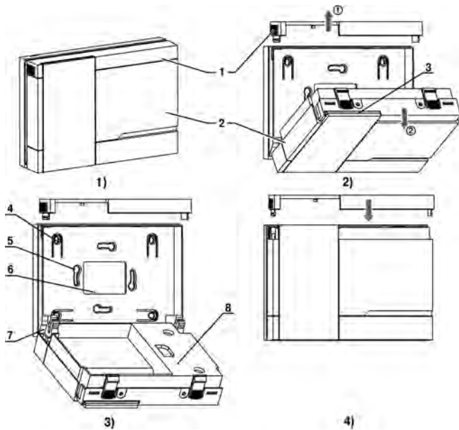
Рисунок 4.3 – Монтаж прибора настенного исполнения N2
