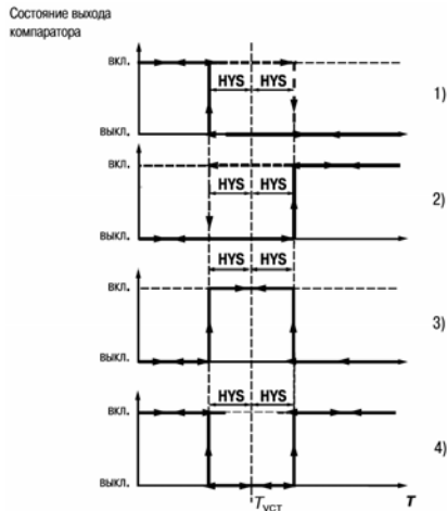
Рисунок 7.9 – Работа регулятора с разными типами логики
