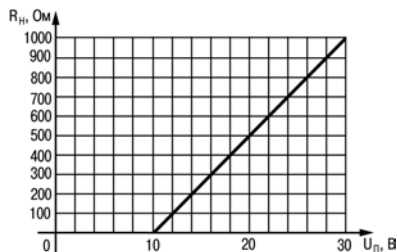
Рисунок 5.18 – График зависимости R_{\text{н}}(U_{\text{н}})
