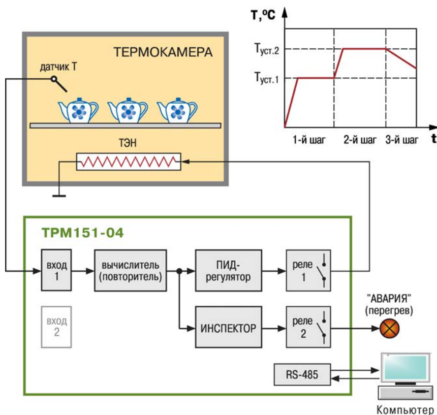
Рисунок 4.6 – Использование 1-канального регулятора TPRM151 04й модификации для поддержания температуры в заданных диапазонах значений при термообработке керамики
