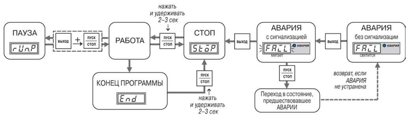
Рисунок 6.4 – Схема переключения состояний прибора
