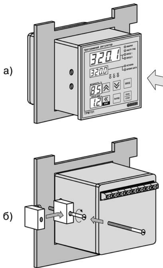
Рисунок 8.2 – Установка прибора щитового крепления
