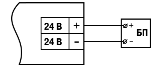
Рисунок 4 – Схема подключения к источнику питания
