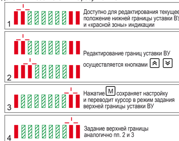
Рисунок 10 – Задание границ сигнализации ВУ и «красной зоны» индикации
