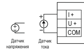
Рисунок 5 – Схемы подключения входных сигналов
