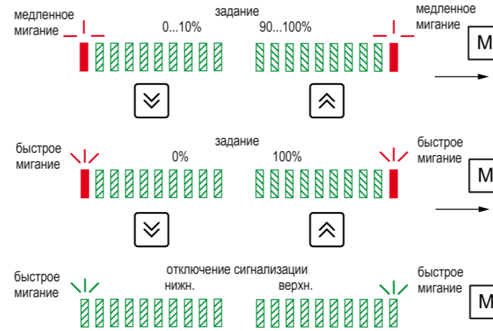
Рисунок 11 – Установка сигнализации на границах измеряемого диапазона
