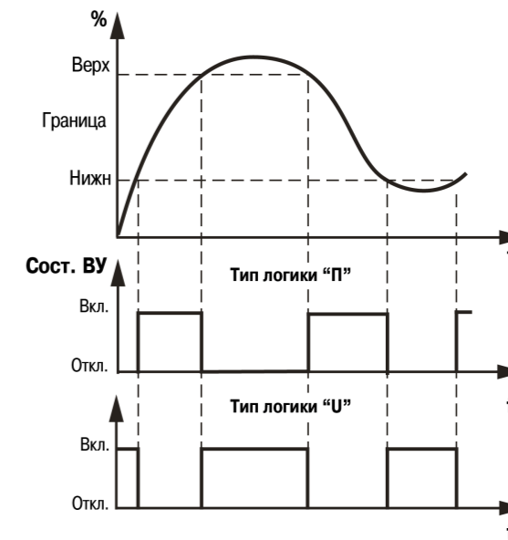
Рисунок 12 – Типы логики работы ВУ
