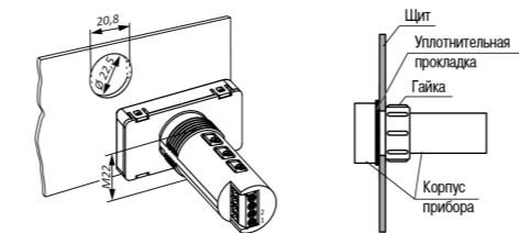
Рисунок 1 – Монтаж прибора щитового крепления
