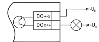
Рисунок 6 – Схема подключения выходного устройства
