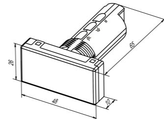
Рисунок 2 – Габаритные размеры корпуса щ9
