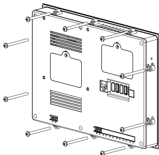
Рисунок 4.3 – Крепление регистратора к щиту
