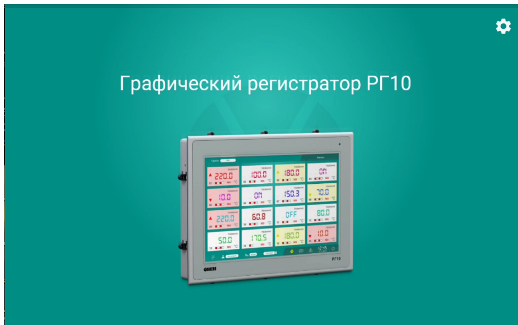
Рисунок 7.1 – Экран приветствия
