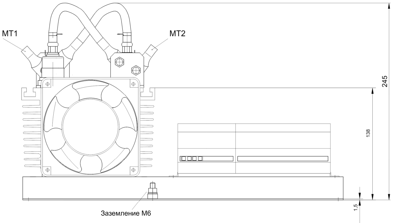
Рисунок 2. Габаритно-установочные размеры
