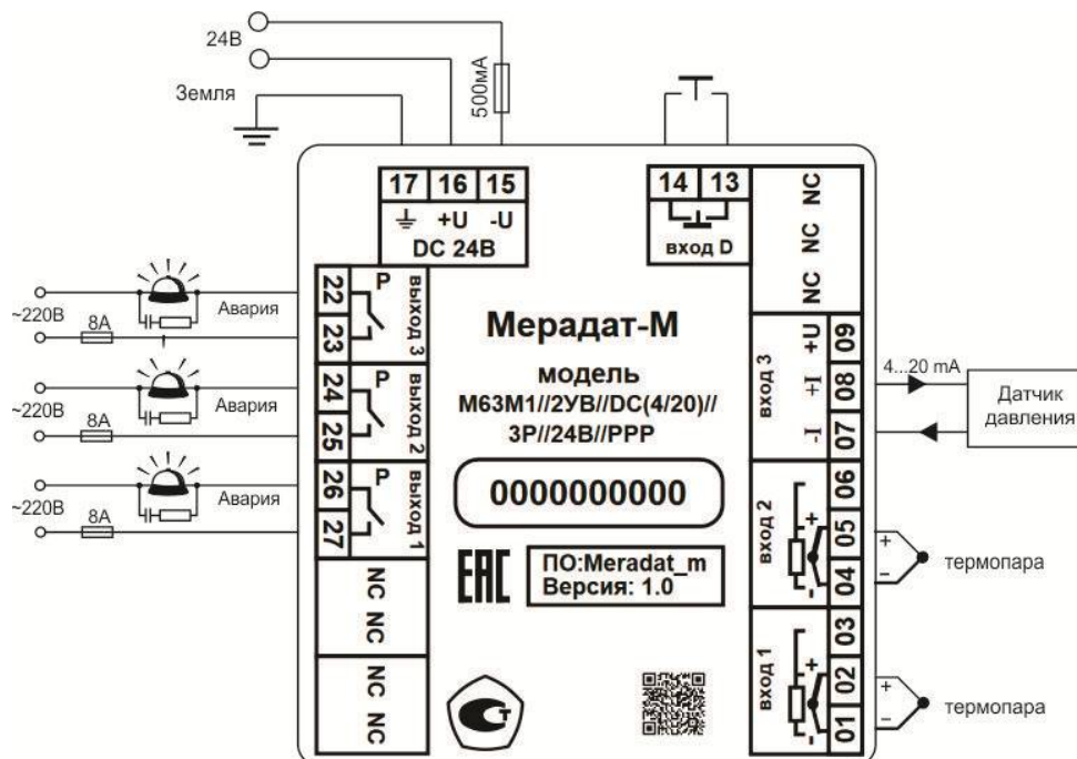
Типовая схема подключения прибора Мерадат-63М1
