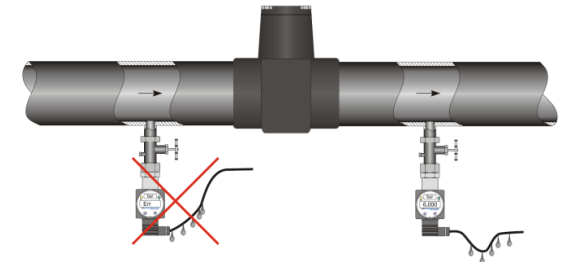
Рисунок 3. Неправильная (слева) и правильная (справа) прокладка кабеля датчика.
