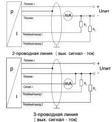
Рисунок 7. Схемы подключения с 1 или 2 релейными выходами DS 200, DS 200P, DS 201, DS 210.
