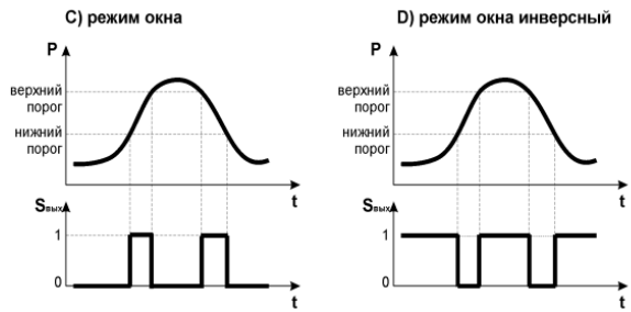
Рисунок С. Режимы работы релейного выхода
