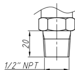
Код N00 (1/2"-14NPT)
