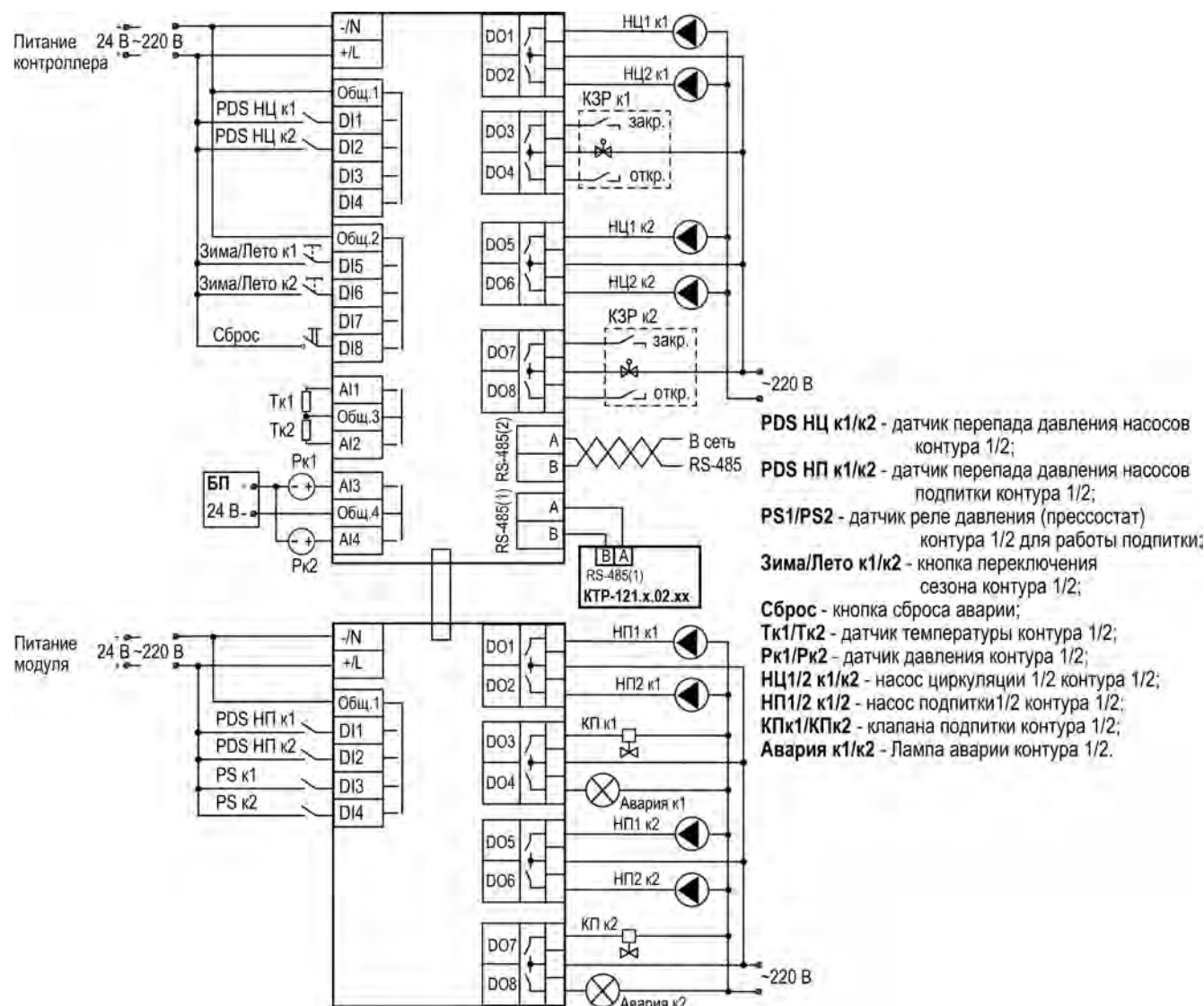
Рисунок 6.4 – Схема подключения KTR-121.03.20 для управления контурами ГВС и отопления с подпиткой
