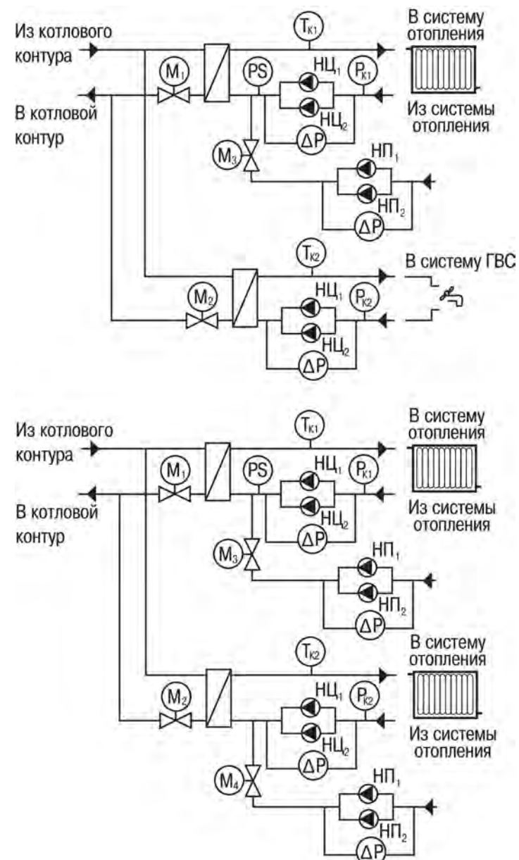
Рисунок 1.2 – Схемы управления контурами ГВС и отопления с подпиткой при использовании КТР-121.03.20 и ПРМ-х.1
