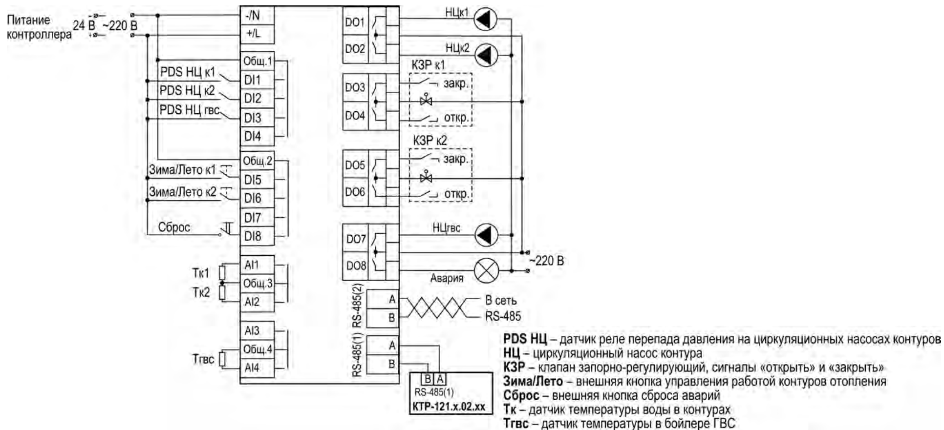
Рисунок 6.4 – Схема подключения KTR-121.03.10 для управления контурами ГВС и отопления
