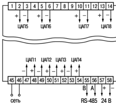
Рисунок Б.5 – Схема размещения ЦАП в приборе модификации ТРМ138В-И
