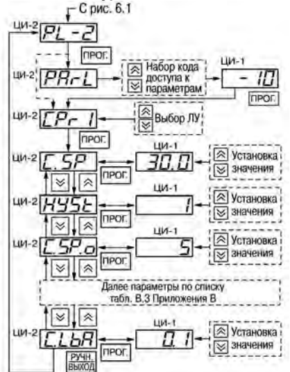
Рисунок 7.4 – Схема установки программируемых параметров на уровне PL-2
