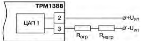
Рис. 3.17. Схема соединения ЦАП с нагрузкой
