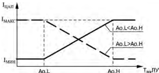
Рисунок 3.12 – Выходные характеристики ЦАП
