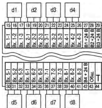
Рисунок Б.4 – Схема размещения симисторных оптопар в приборе модификации ТРМ 138В-С
