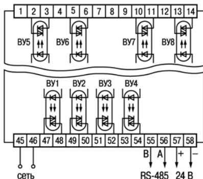
Рисунок Б.4 – Схема размещения симисторных оптопар в приборе модификации ТРМ 138В-С
